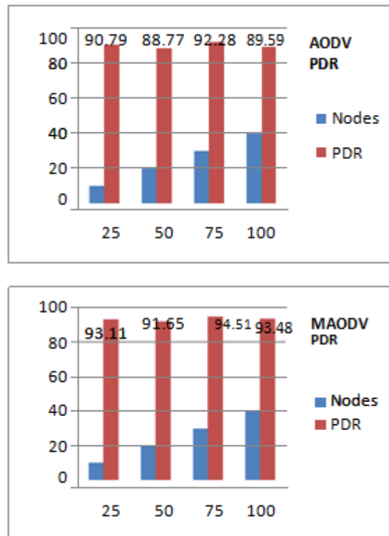
Fig: PDR Result
